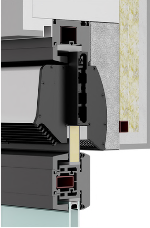
Yatay Sercair - Üst Sabit Doğrama İç (Orta Kayıt) - Perspektif
