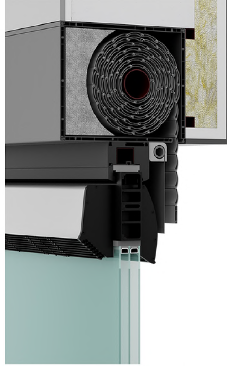
Doğrama İç Yatay Sercair - Monoblok Panjur Montajı Detayı - Perspektif
